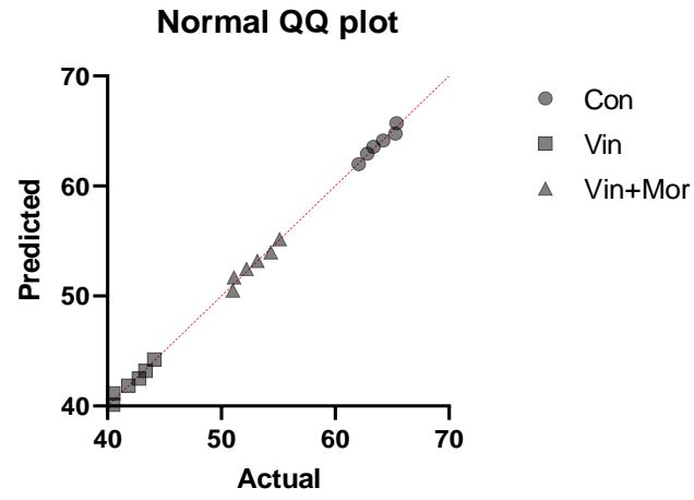
Q-Q plots for Fig. 2A
