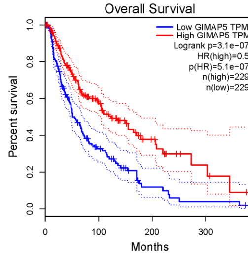
GIMAP5
